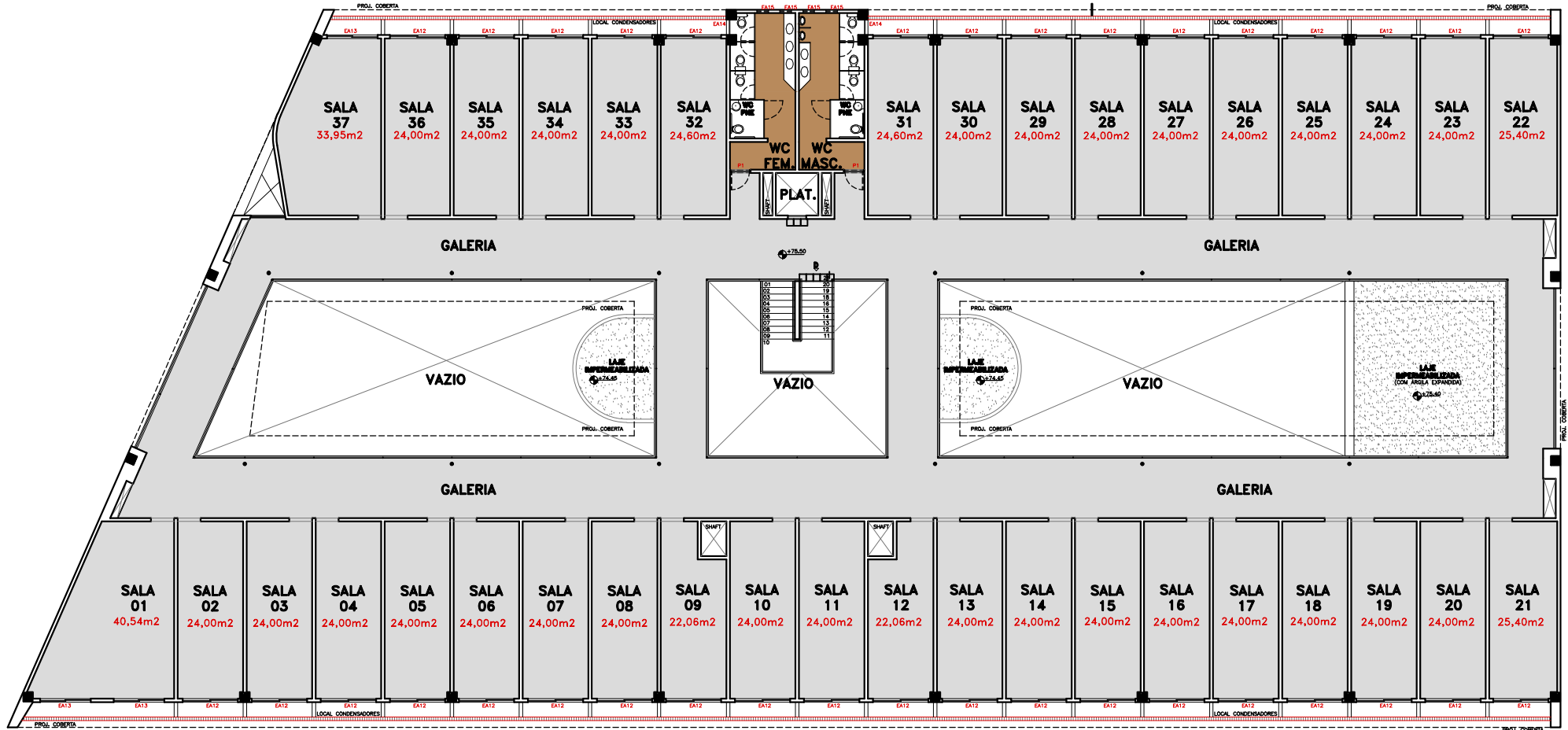
PLANTA BAIXA - 1º PAV.
